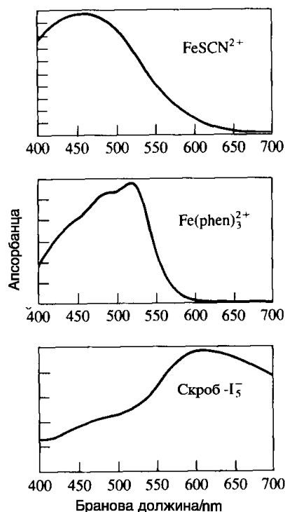
Слика 12. Спектри на комплекси со пренос на електрони во видливото подрачје
