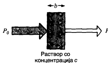
Слика 5. Намалување на интензитетот на зрачењето како последица на апсорпција од страна на конституентите на растворот
