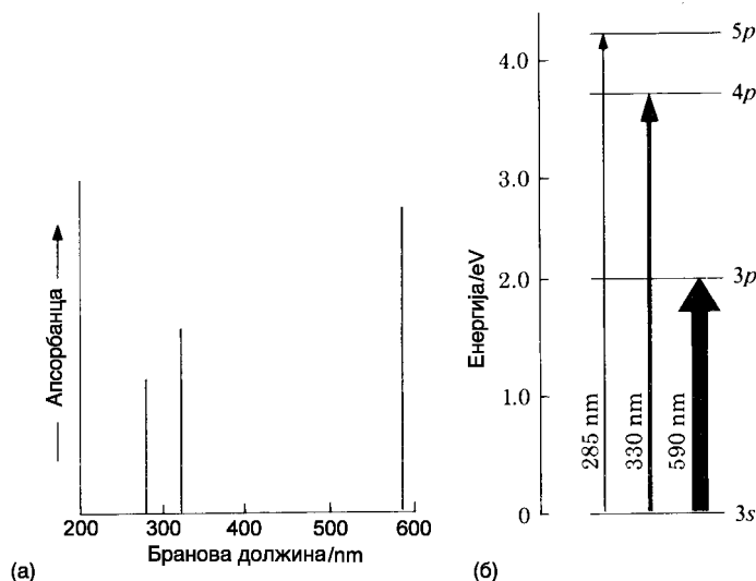
Слика 3. а-Апсорпционен спектар на гасовит натриум. б-дијаграм на енергетските нивоа на натриумот со приказ на електронските премини и енергетските нивоа.
