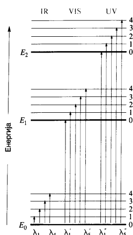
Слика 4. Дијаграм на електронски енергетски нивоа: E_1 , E_1 и E_2 (во рамките на кои може да се видат и вибрациони нивоа: 0, 1, 2, 3 и 4) и премини помеѓу нив.
